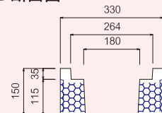
B-B'断面図
