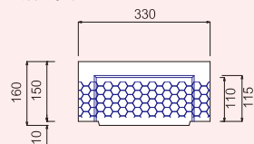
A-A'断面図
